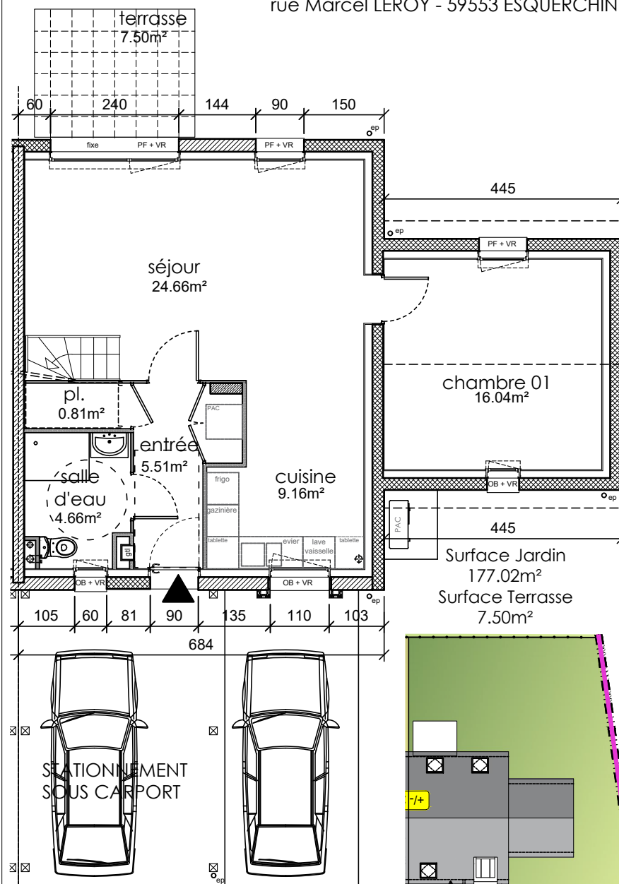
Rez-de-Chaussée
