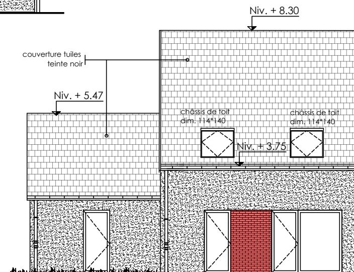
Façade Arrière
