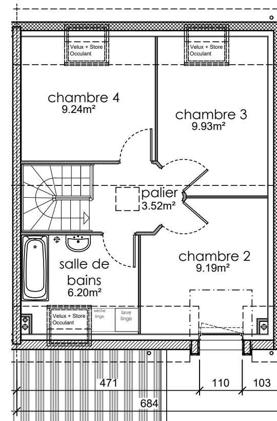
Etage
