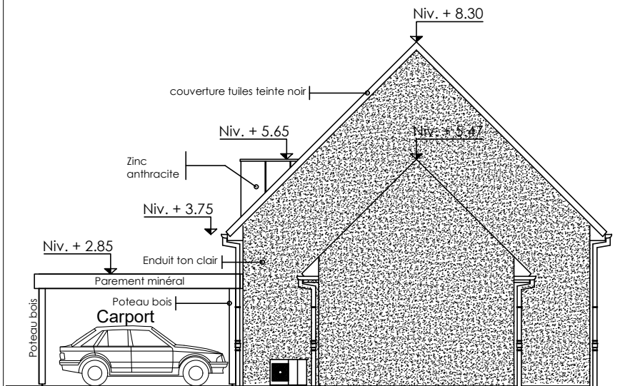
Pignon Droit
